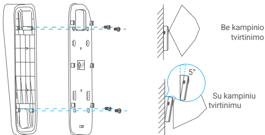
Pav.2 Kampinis tvirtinimas
