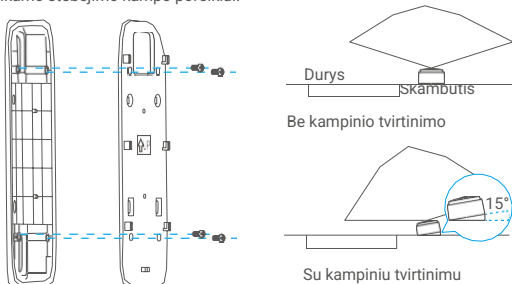
Pav.1 Kampinis tvirtinimas
